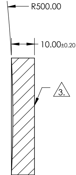
SECTION A-A
