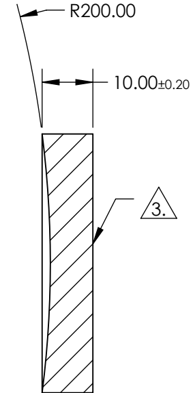
SECTION A-A
